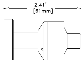
Mini Conflat™ (HPM-2002s-03)
